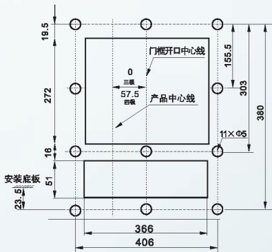
固定式断路器用门框柜上开孔尺寸 SW8-3200固定式
