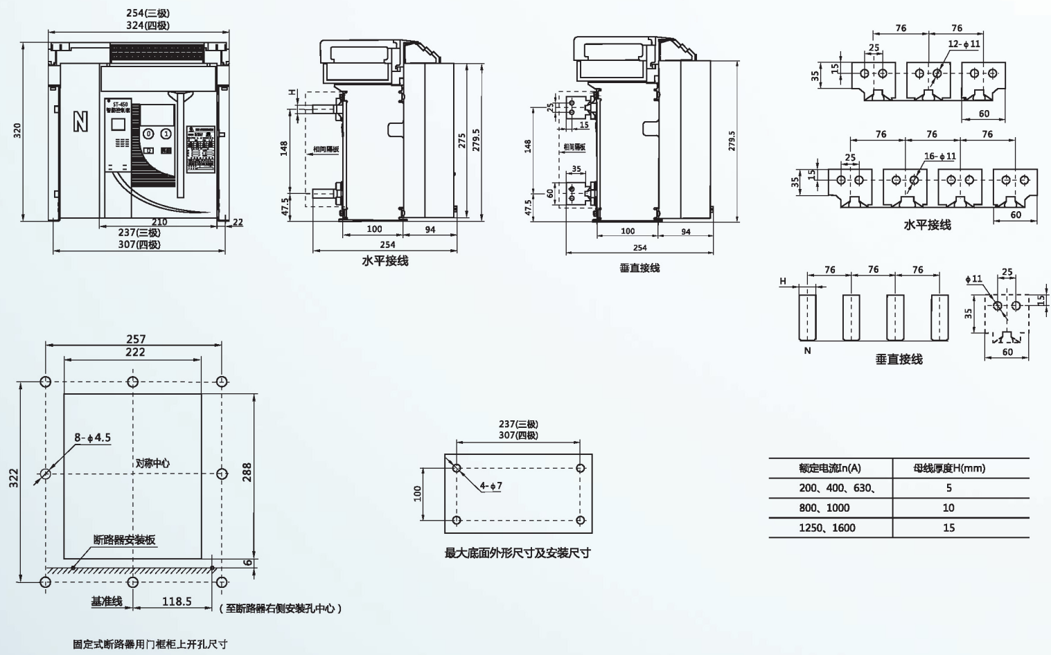
SW8-1600固定式
