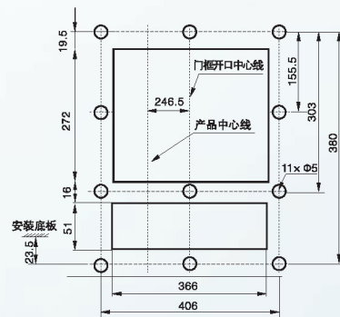
抽屉式断路器用门框柜上开孔尺寸
