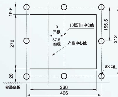
固定式断路器用门框柜上开孔尺寸
