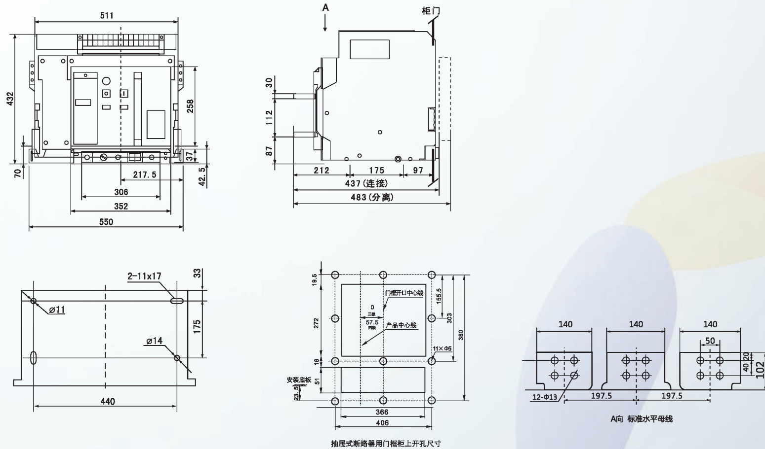
SW8-4000抽屉式(柜II扩容)
