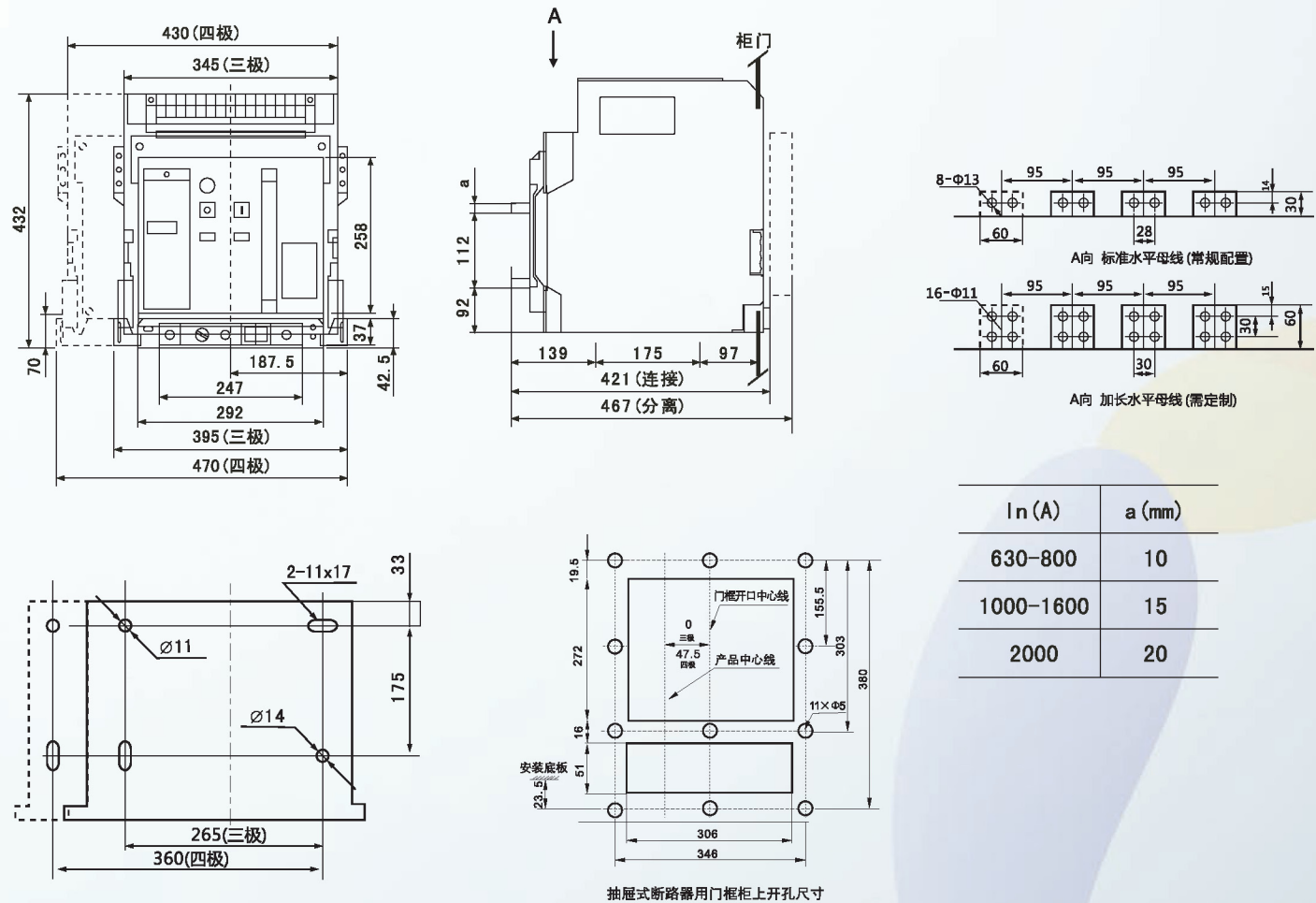
SW8-2000抽屉式
