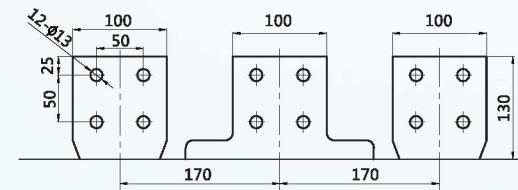
A向 标准水平母线
