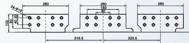
SW8-6300/3抽屉式母线
