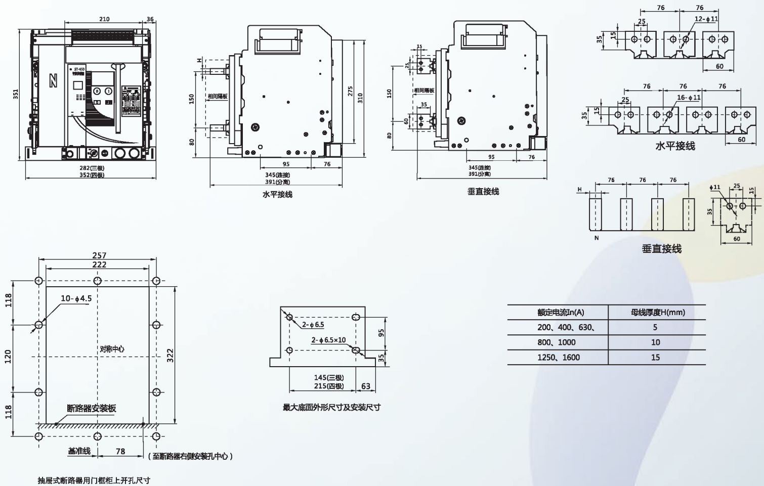
SW8-1600抽屉式
