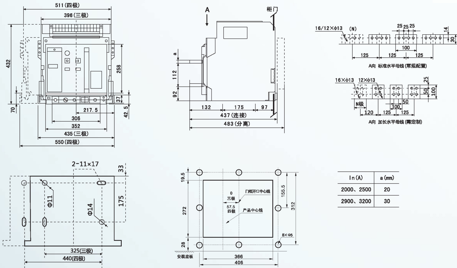
抽屉式断路器用门框柜上开孔尺寸
