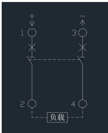
接线图 1
