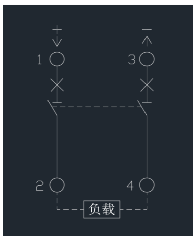
接线图 1
