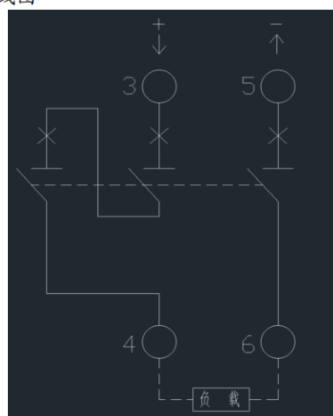
接线图 2
